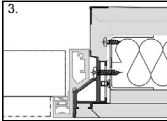
3. Trockenbau, durch die Leibung öffnend
