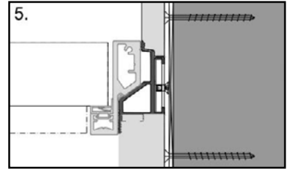
5. Montage in der Leibung
