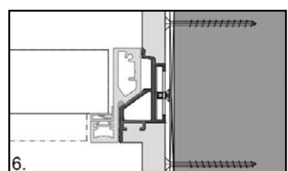
6. Montage in der Leibung
