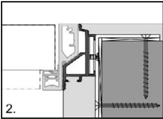
2. Mauerwerk, herkömmlich öffnend
