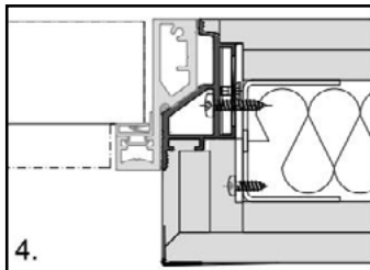
4. Trockenbau, herkömmlich öffnend
