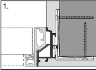
1. Mauerwerk, durch die Leibung öffnend
